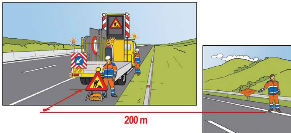
Figura 23 bis – Chiusura della corsia di emergenza: installazione del segnale lavori
