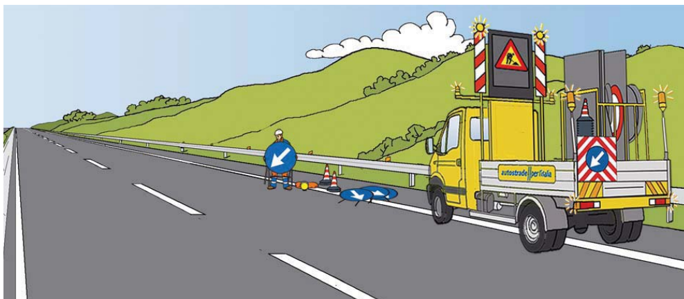
Figura 49 – Chiusura della corsia di marcia: scarico della segnaletica di testata sul margine destro
